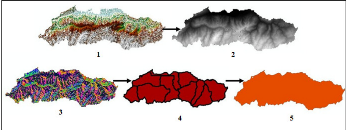
Şekil 2.4. Çalışma alanı sınırlarının hidroloji analizi ile belirlenmesi (Aydın ve diğ. 2012). (1:Yüzey hazırlığı aşaması, 2:Akış yönünün belirlenmesi, 3:Drenaj ağlarının oluşturulması, 4: Alt havza sınırlarının belirlenmesi, 5: Havza sınırının belirlenmesi).
