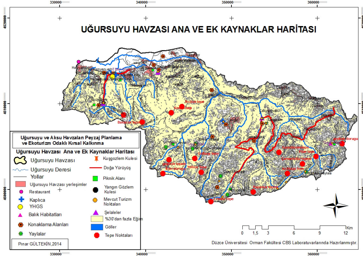
Şekil 3.36. Uğursuyu Havzası ana ve ek kaynaklar akıştırma haritası
