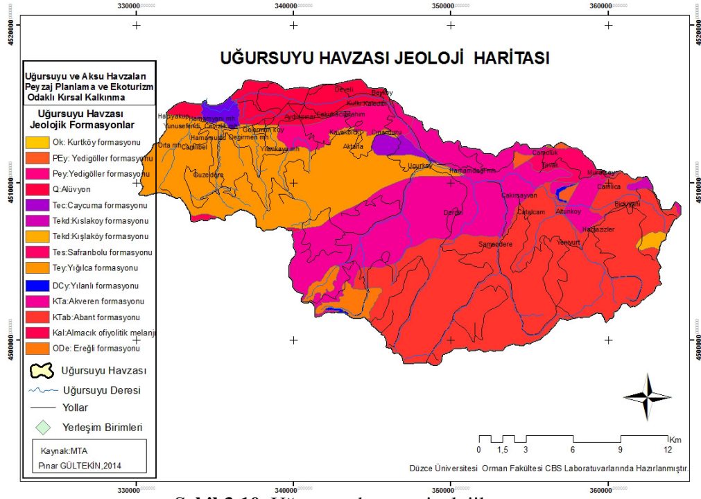
Şekil 3.10. Uğursuyu havzası jeolojik yapı
