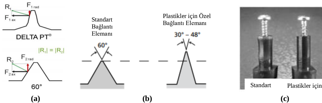
Şekil 1. a) Dişli profili açısının bir fonksiyonu olarak elde edilen kuvvetler, b) Özel vida ve standart vida dişi profili, c) Özel vida ve standart vida dişi tasarımlarının ince duvarlı bölgelerde nasıl çalışabileceğini gösteren örnek resim [4].
