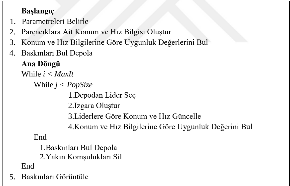
Şekil 6.3. HCA-RGO sözde kod.
