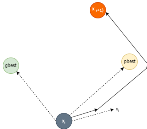
Şekil 3.1. PSO parçacık konum ve hız güncelleme.
