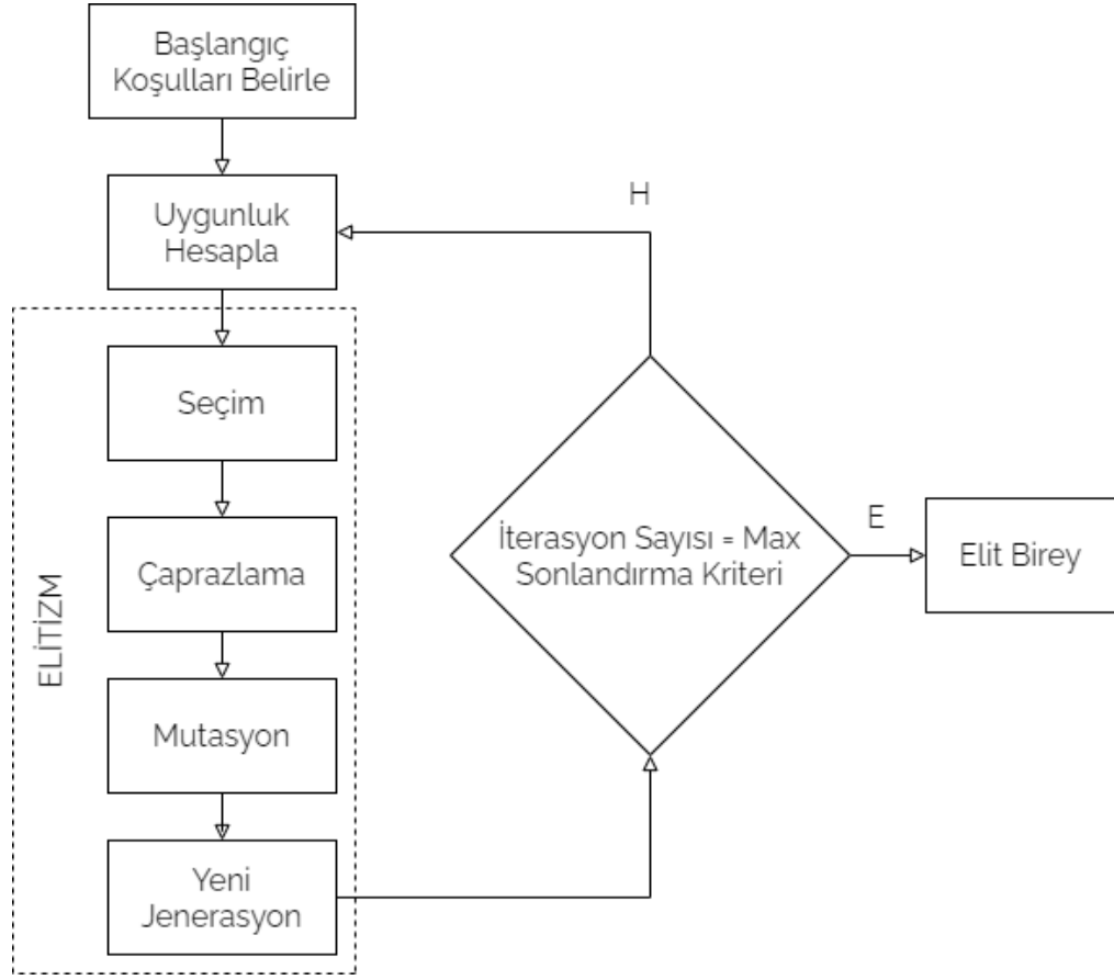
Şekil 3.8. Genetik Algoritma akış diyagramı.
