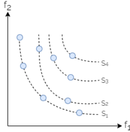
Şekil 5.4. Sıralama örneği.
