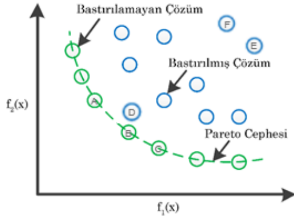
Şekil 5.1. Baskınlık ilişkisi.
