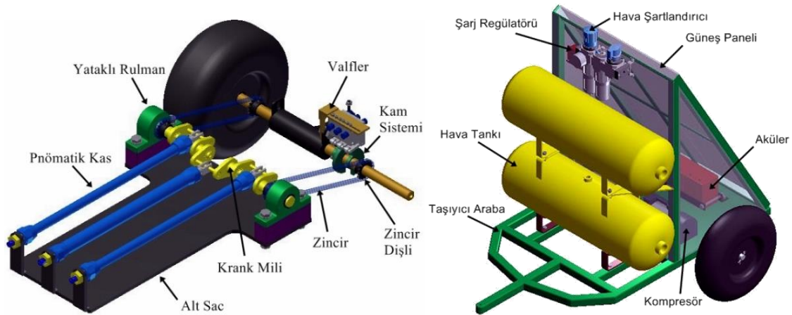
Şekil 2. Hareket ve güç ünitesi
