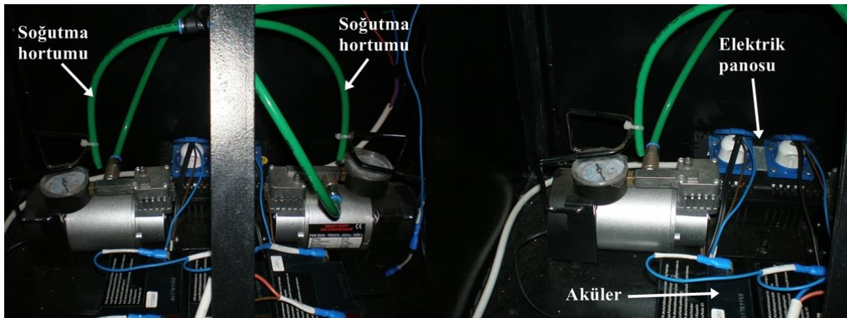
Şekil 7. Soğutma sistemi ve elektrik panosu
