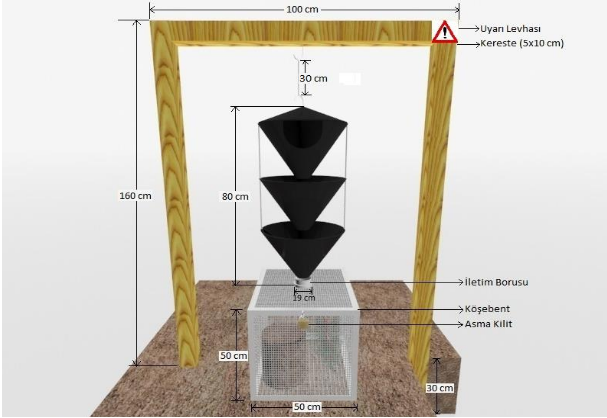
Şekil 1. Böcek toplamak için geliştirilen kafes ve bölümleri
