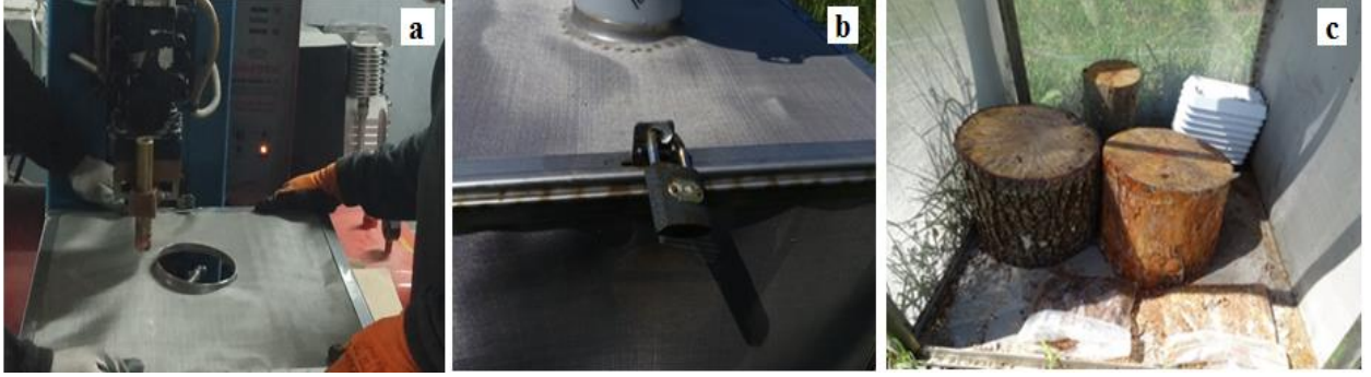
Şekil 2. a) Böcek toplama kafesinin imalatı b) Kafes güvenlik aparatı c) Kafes içerisine konulan materyaller
