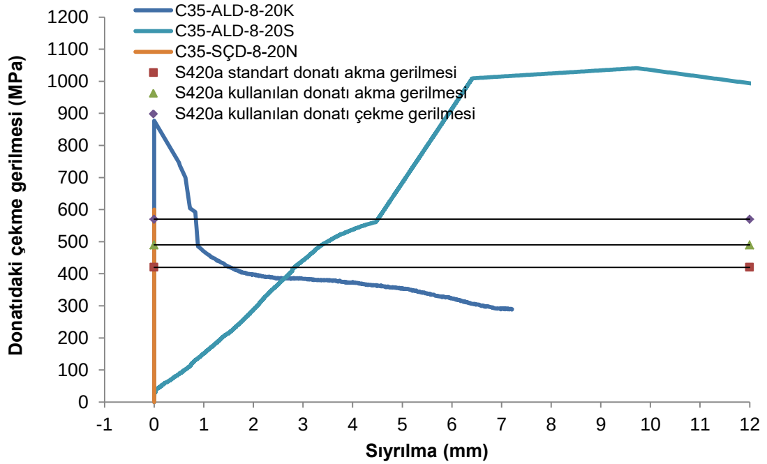
Şekil 6.9. C35 beton-8 mm donatı çapı ve 20Φ kenetlenmede aramid lifli donatı gerilme-sıyrılma ilişkisi.
