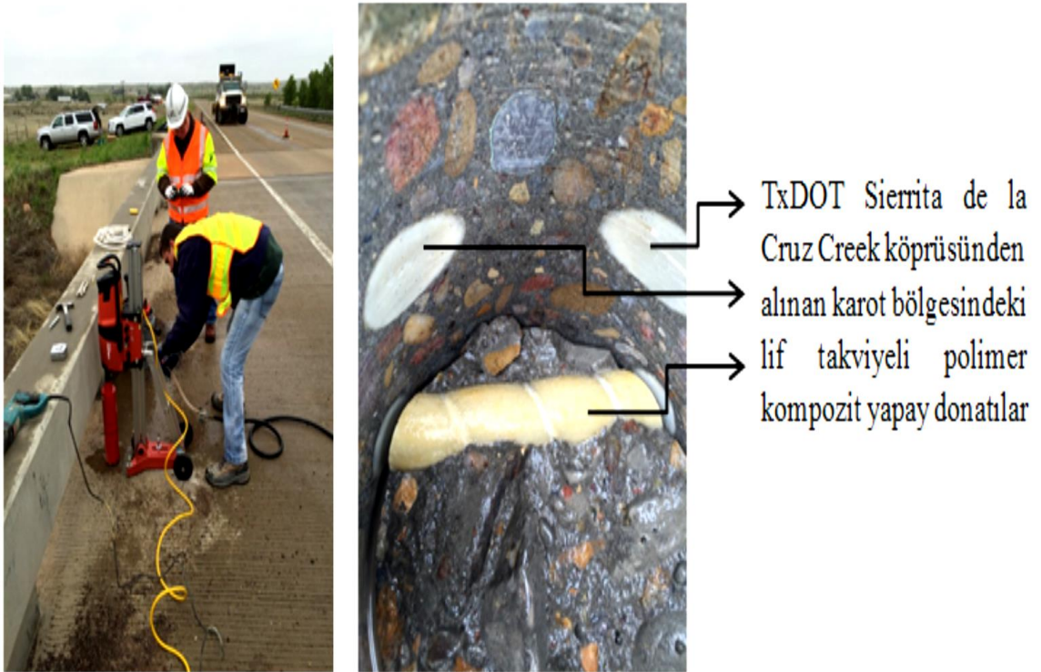
řekil 1.12. Lif takviyeli donatıların durabilite kabiliyeti [14].
