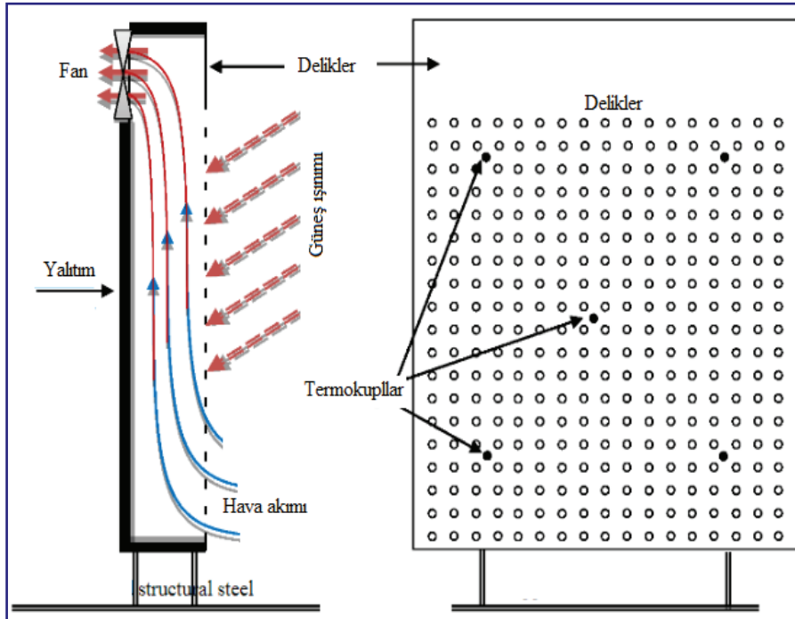
Şekil 9. Analiz edilen deneysel sistem [13]
