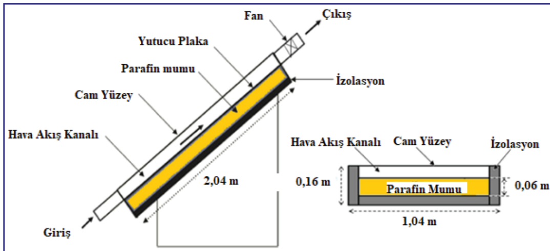
Şekil 7. Faz değişkenli havalı güneş kollektörünün şematik gösterimi ve boyutları [11]
