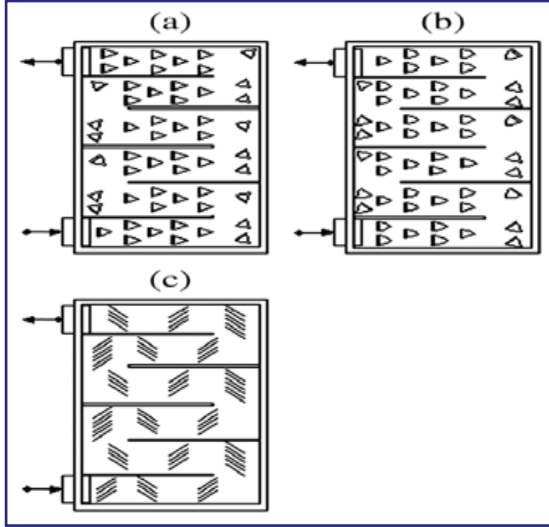
Şekil 5. Farklı tasarımlardaki emici yüzeyli havali kolektörler (a) Üçgen (b) Yaprak (c) Dikdörtgen [4]
