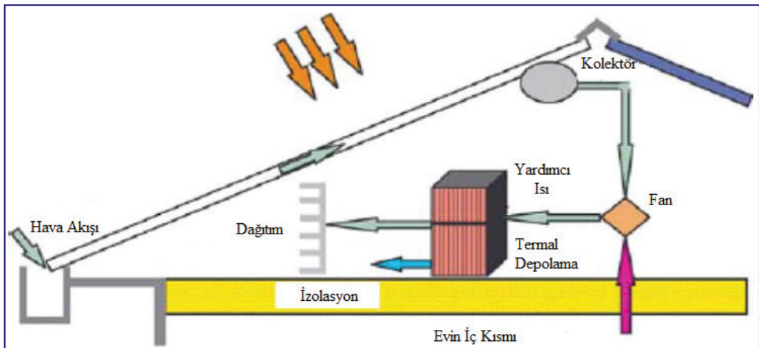
Şekil 6. Depolama ünitesi tavana entegre havali güneş enerjisi ısıtma sistemi [9]
