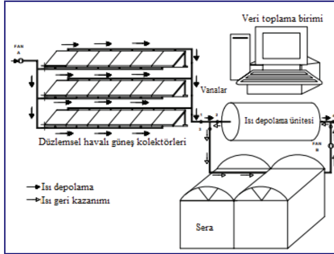
Şekil 6. Depolama malzemesi ile hava ısıtıcı görünümü [10]
