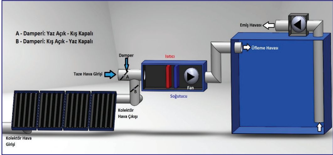
Şekil 11. Taze havalı iklimlendirme sistemi örnek uygulaması
