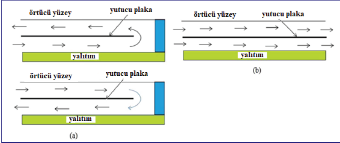
Şekil 2. İki geçişli havalı güneş kolektörü (a) Karşı akış (b) Paralel akış [4]
