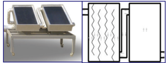
Şekil 4. Zigzag ve düz emici yüzeyli havalı bir güneş kolektörü [6]
