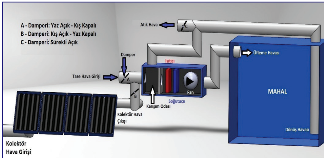
Şekil 10. Karışım havalı iklimlendirme sistemi örnek uygulaması
