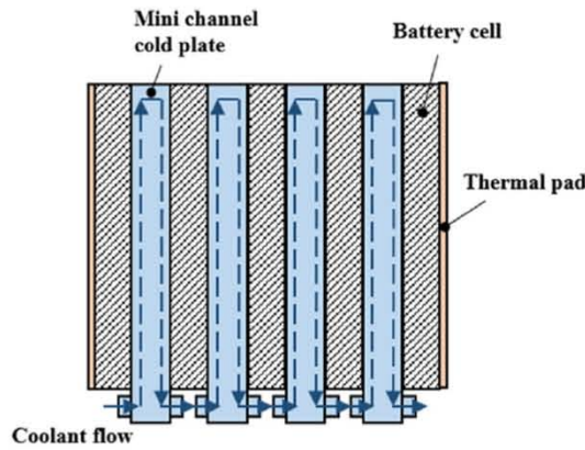
Fig. 9 Mini channel cold plate cooling [56]
