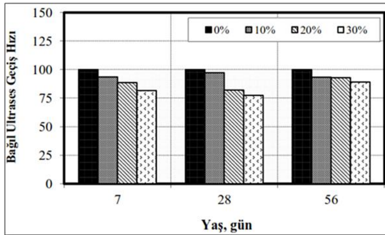
Şekil 4. Harç numunelerinin bağıl ultrases geçiş hızı değerleri [19]
