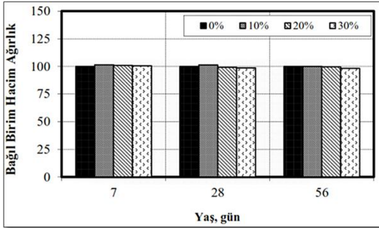
Şekil 3. Harç numunelerinin bağıl birim hacim ağırlık değerleri [19]
