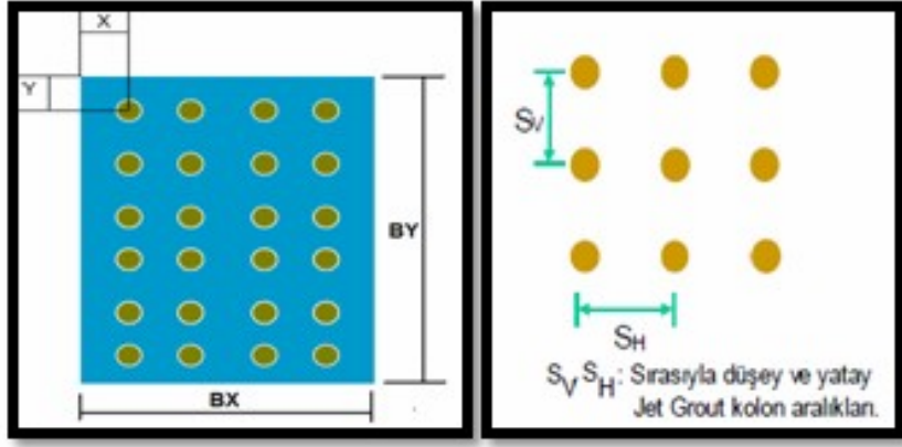
Şekil 10. Jetgrout Kolon Aralıkları ve Mesafeleri
